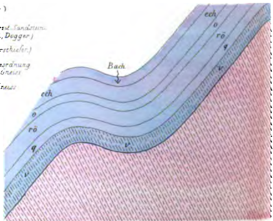
Fig. 7. Überspringen der Schieferung vom Glimmerschiefer auf den Verrucano ob der Spitzgrassenplangge am Fuss des Schlawbergs
